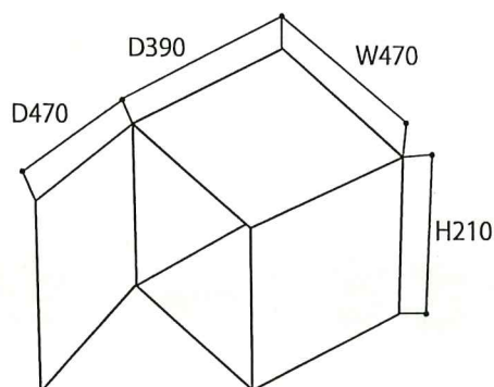
内寸法
